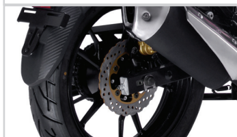
Δίσκοι μαργαρίτα με διπίστονες δαγκάνες και σύστημα πέδησης CBS
